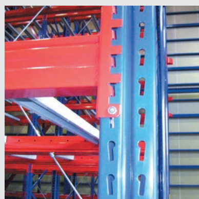
中国製パレットラック
